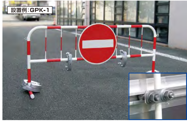
設置例:GPK-1 GPK-1の標識固定には、アルミフラットバー(別売)を使用しております。アルミフラットバーはφ13のバリケードに使用します。
