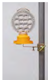
取付事例③ アルファ専用 支柱取付ベース (φ50mm用) DSK-A3 531533
